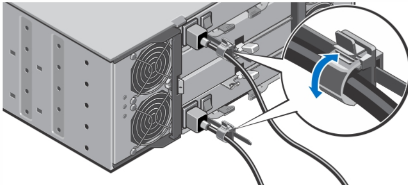
Abbildung 5. Stromkabel befestigen
